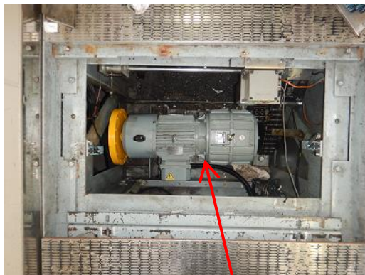
巻上機
